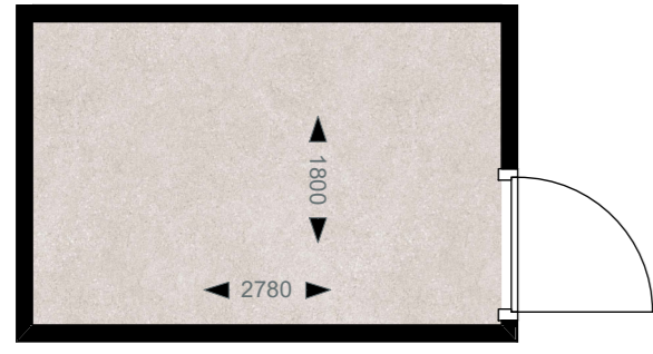
berging - schaal 1:50
